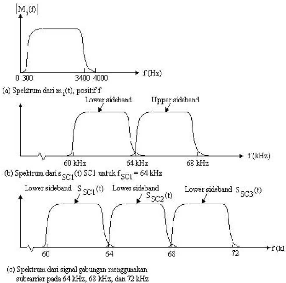
Gambar 6.5. FDM dari tiga sinyal band suara.
