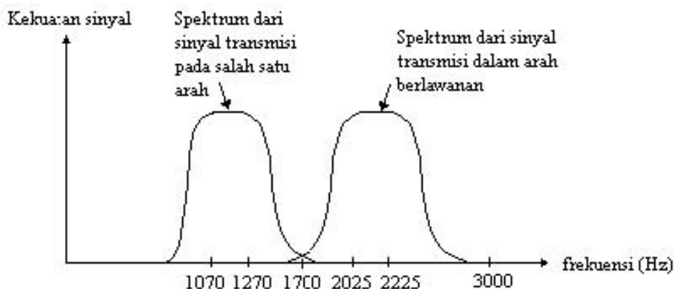
Gambar 3.7. Transmisi FSK full-duplex pada line voice-grade
