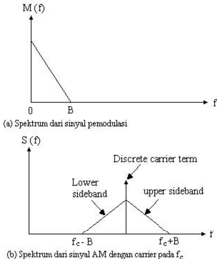
Gambar 3.18. Spektrum dari sebuah sinyal AM.
