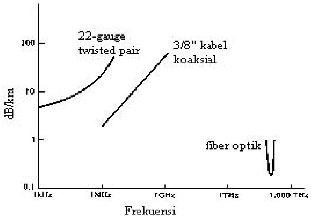
Gambar 2.18 Attenuasi / pelemahan Pada Media Transmisi Guided
