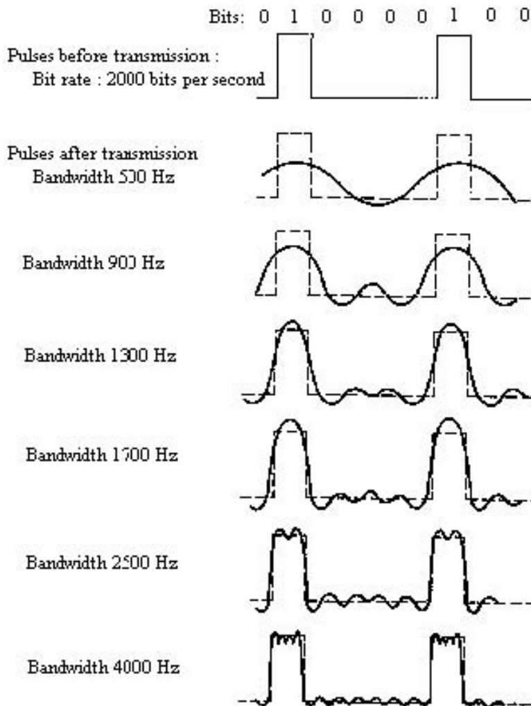
Gambar 2.9. Efek dari bandwidth pada suatu sinyal digital
