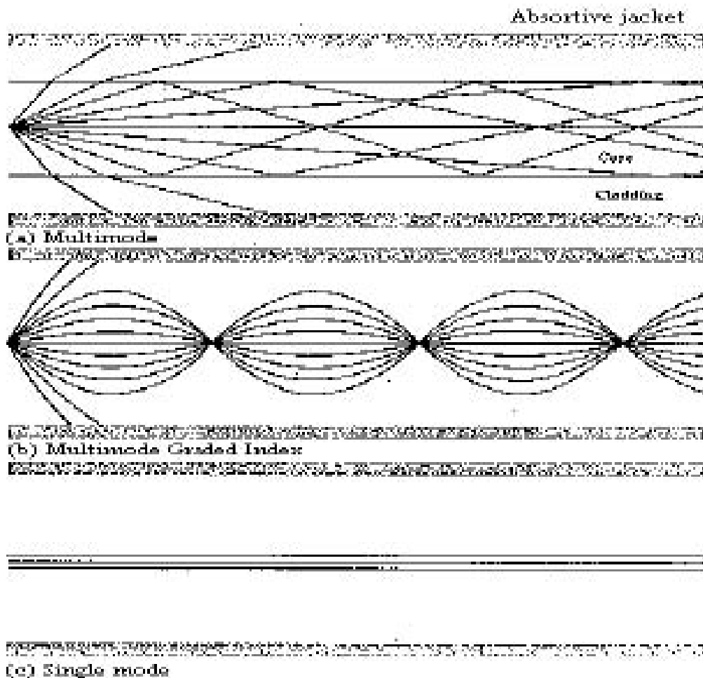
Gambar 2.22. Mode Transmisi dari Fiber Optik
