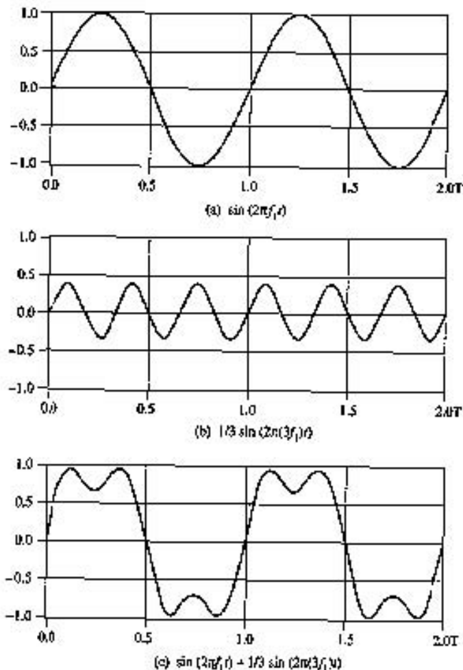
Gambar 2.5. Penjumlahan dari komponen frekuensi ( T= 1/f_1 ).
