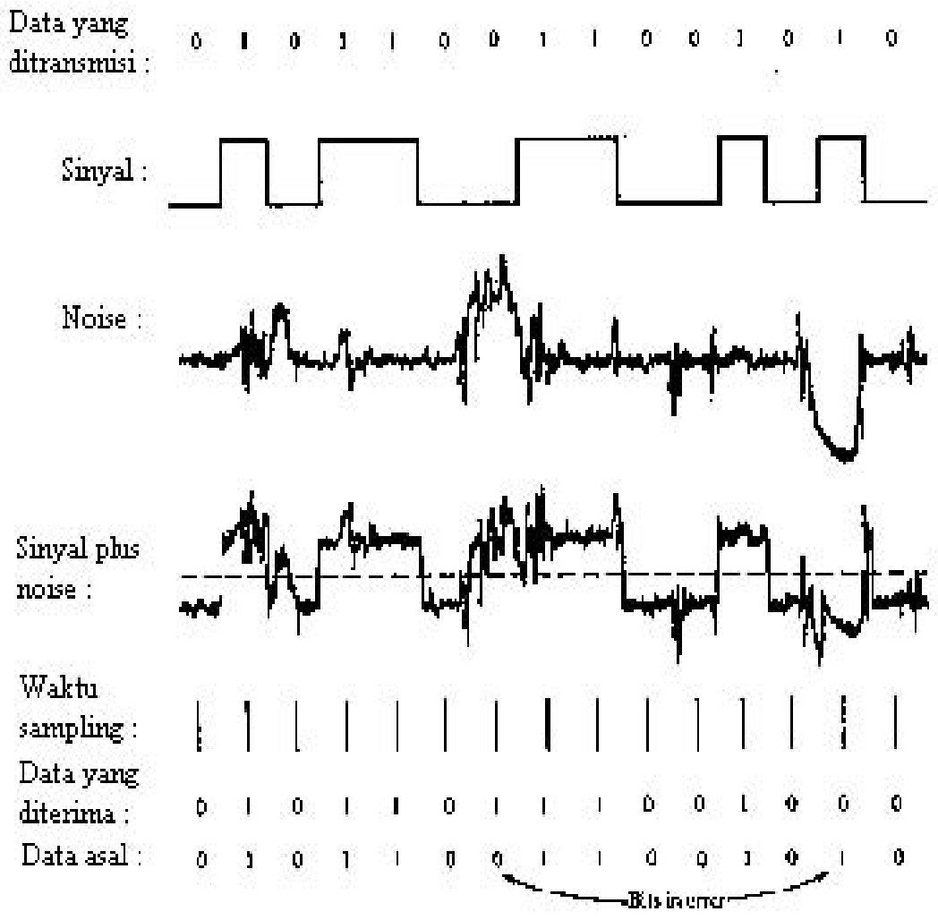
Gambar 2.15. Efek Dari Noise Pada Sinyal Digital
