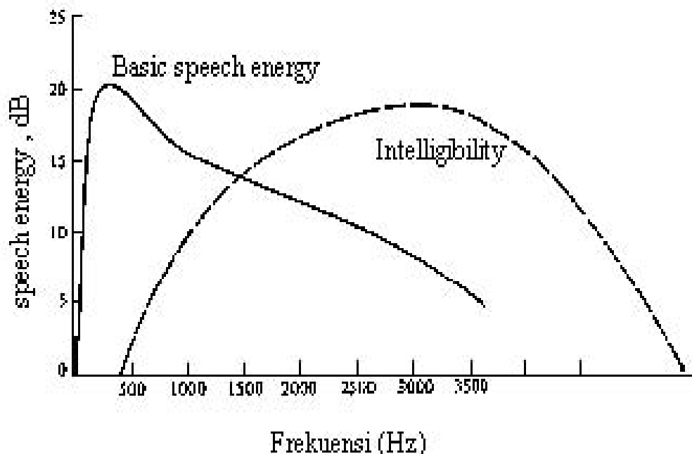
Gambar 2.10. Spektrum akusisi untuk speech
