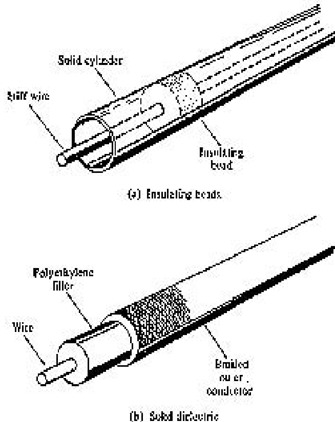
Gambar 2.20 Konstruksi Kabel Koaksial
