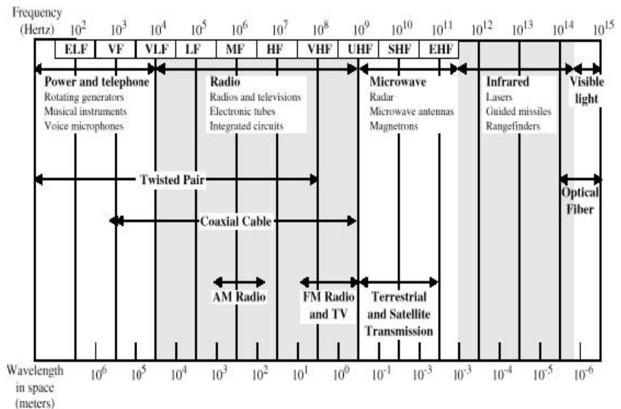
Gambar 2.17. Spektrum elektromagnetik
