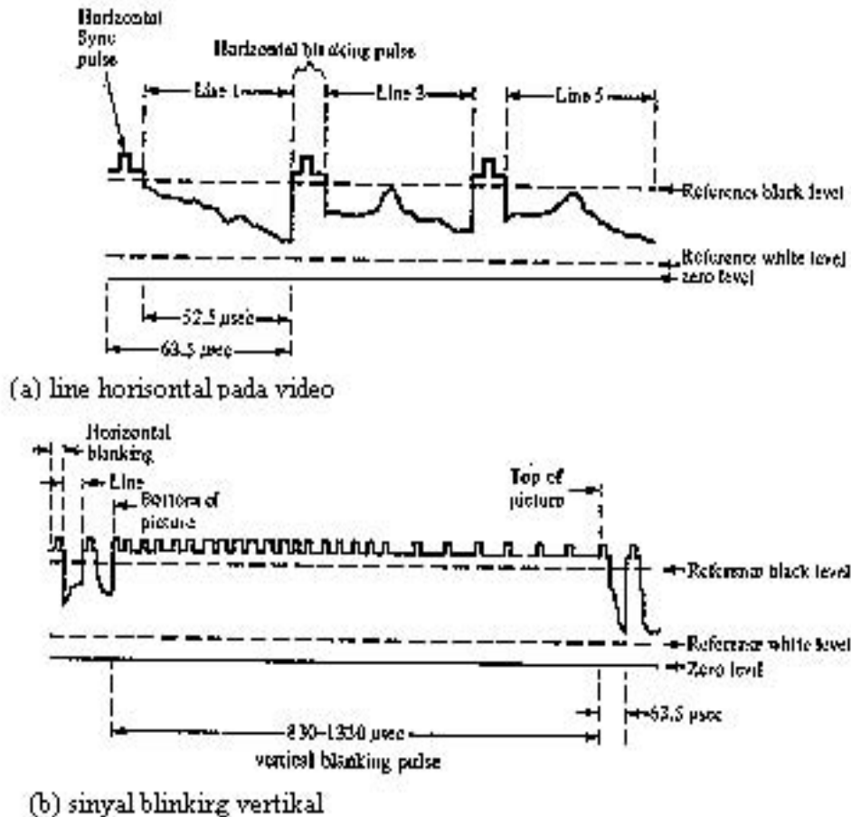
Gambar 2.12. Sinyal video (skala yang berbeda untuk a dan b)
