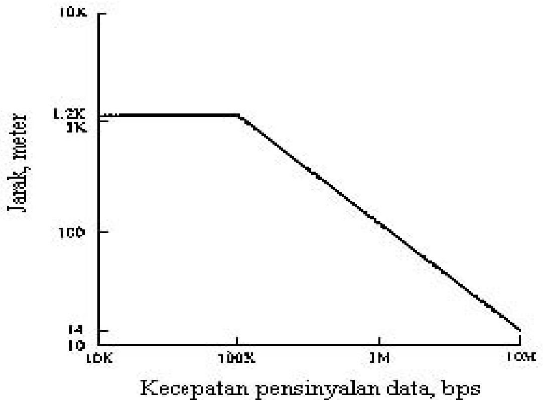
Gambar 2.19. Panjang Kabel Twisted Pair VS Data Rate Untuk Keseimbangan Transmisi
