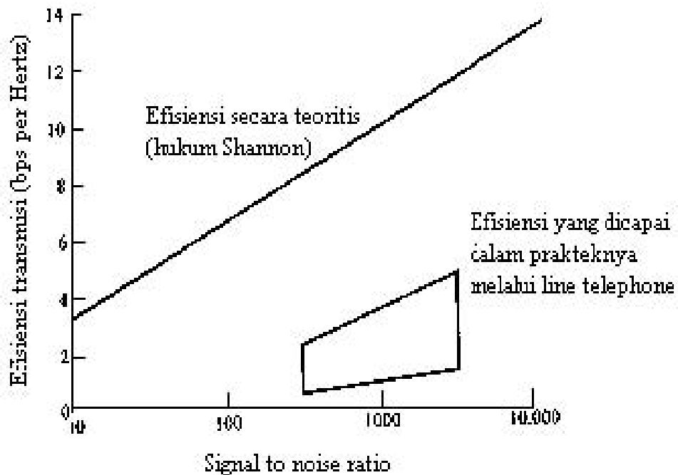
Gambar 2.16. Efisiensi Transmisi Secara Teoritis dan Sebenarnya
